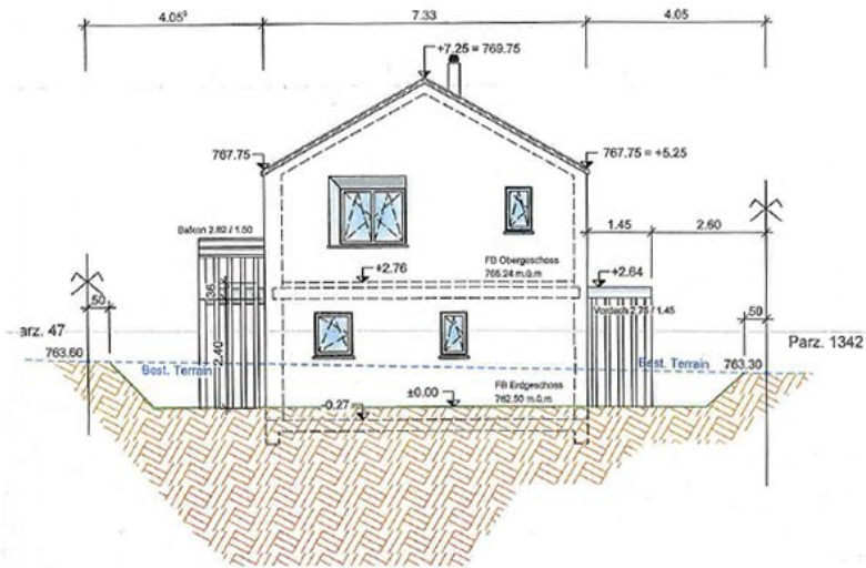
Ansicht Ost Haus 2 1:100
