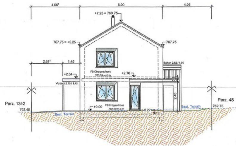
Ansicht West Haus 2 1:100
