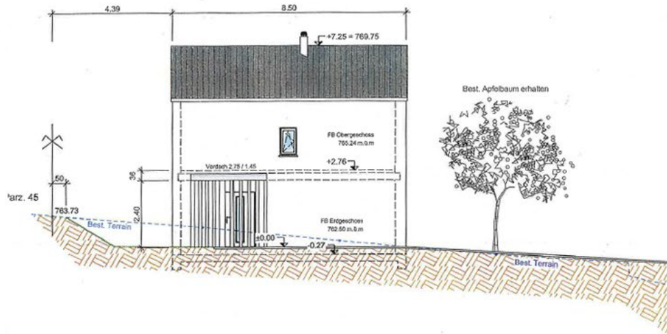
Ansicht Nord Haus 2 1:100
