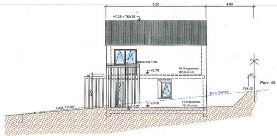
Ansicht Süd Haus 2 1:100
